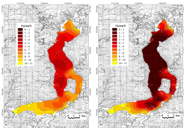
Figura 5. Distribuzione spaziale della concentrazione media di ozono disciolto nell'atmosfera (a) e negli ultimi 10 metri in prossimità del fondo (b).
